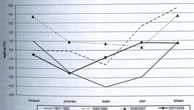
Vysoké nad Jizerou - průměrné měsíční teploty vzduchu ve vybraných zimních obdobích
