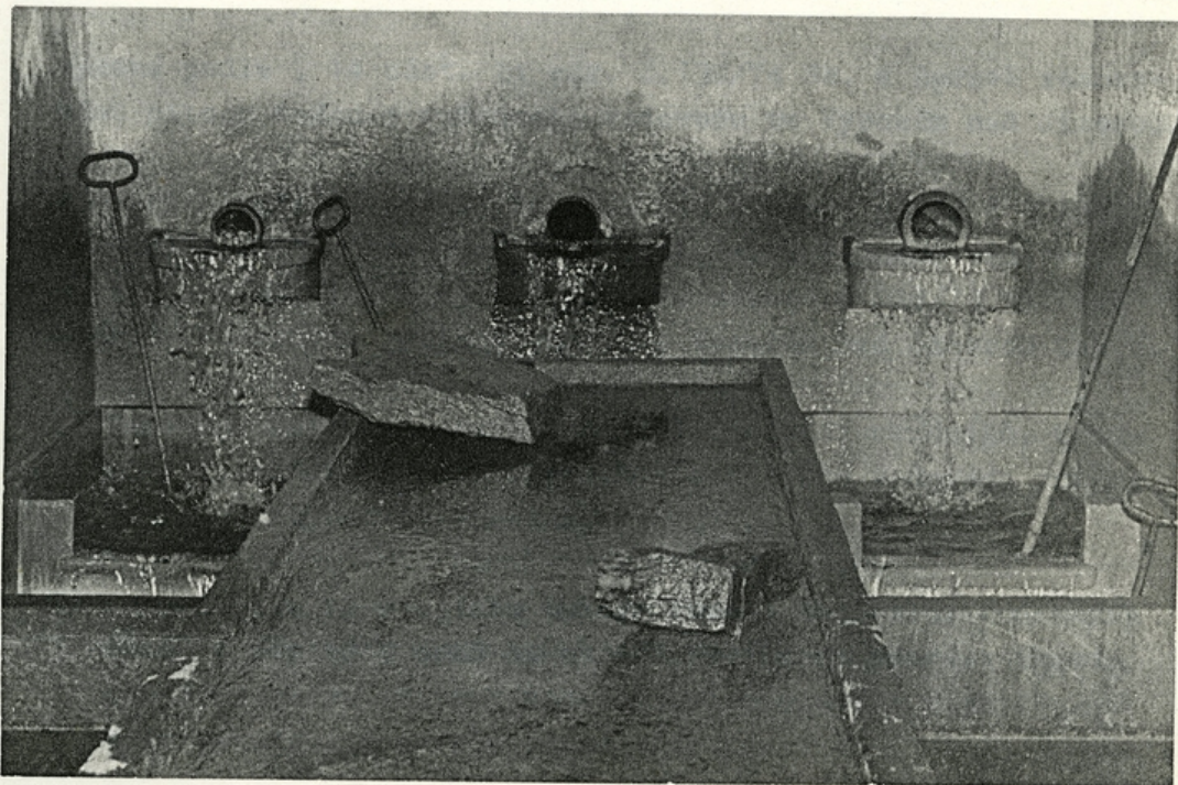
HLAVNÍ SBĚRNA - počátek gravitačního vodovodu Rejdice - Vysoké
